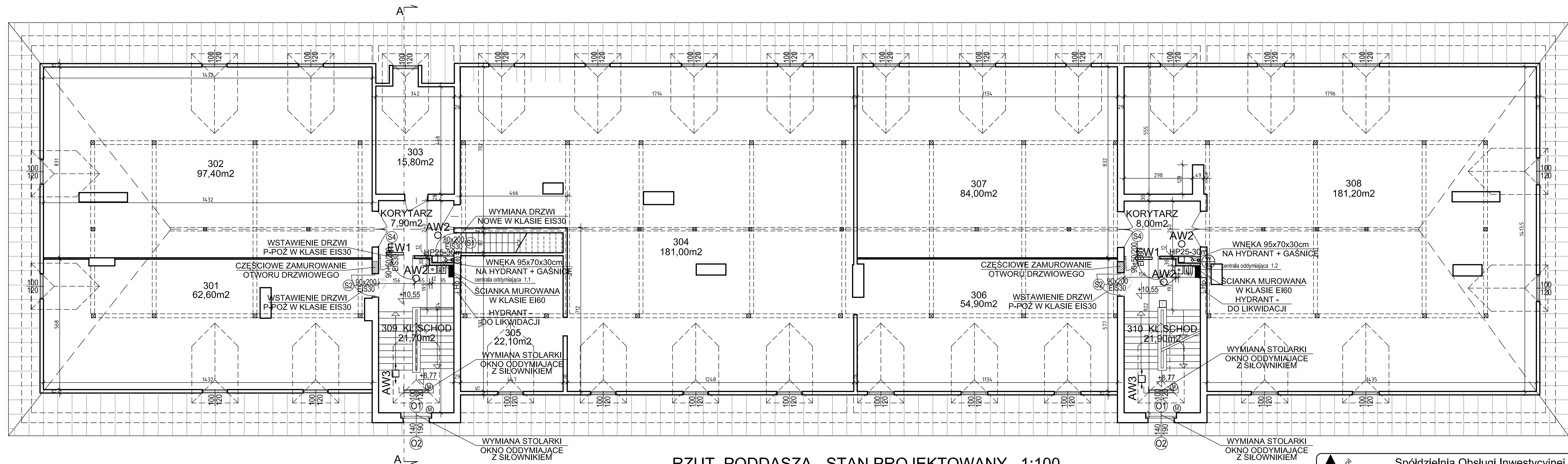
RZUT PODDASZA - STAN PROJEKTOWANY 1:100 BUDYNEK "B"
