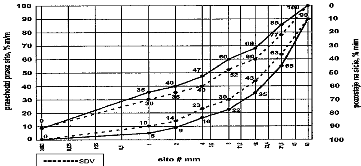
Rys. 1a. Krzywe graniczne uziarnienia mieszanki kruszywa niezwiązanego 0/63 mm do warstw podbudowy zasadniczej
