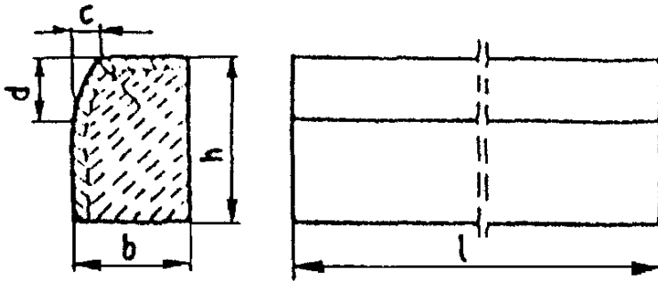
Rys. 1. Wymiarowanie krawężników
