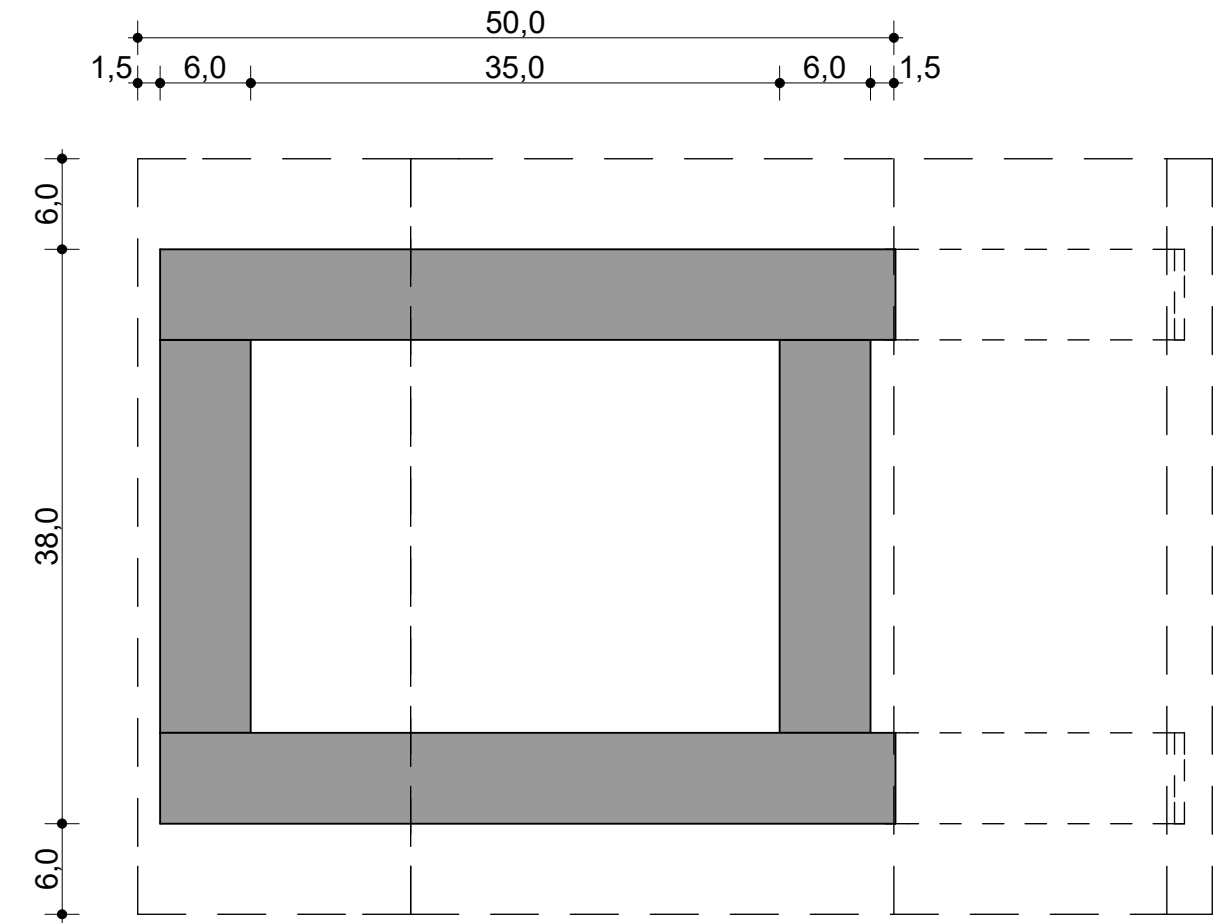
WIDOK PODSTAWY POD SIEDZISKIEM
