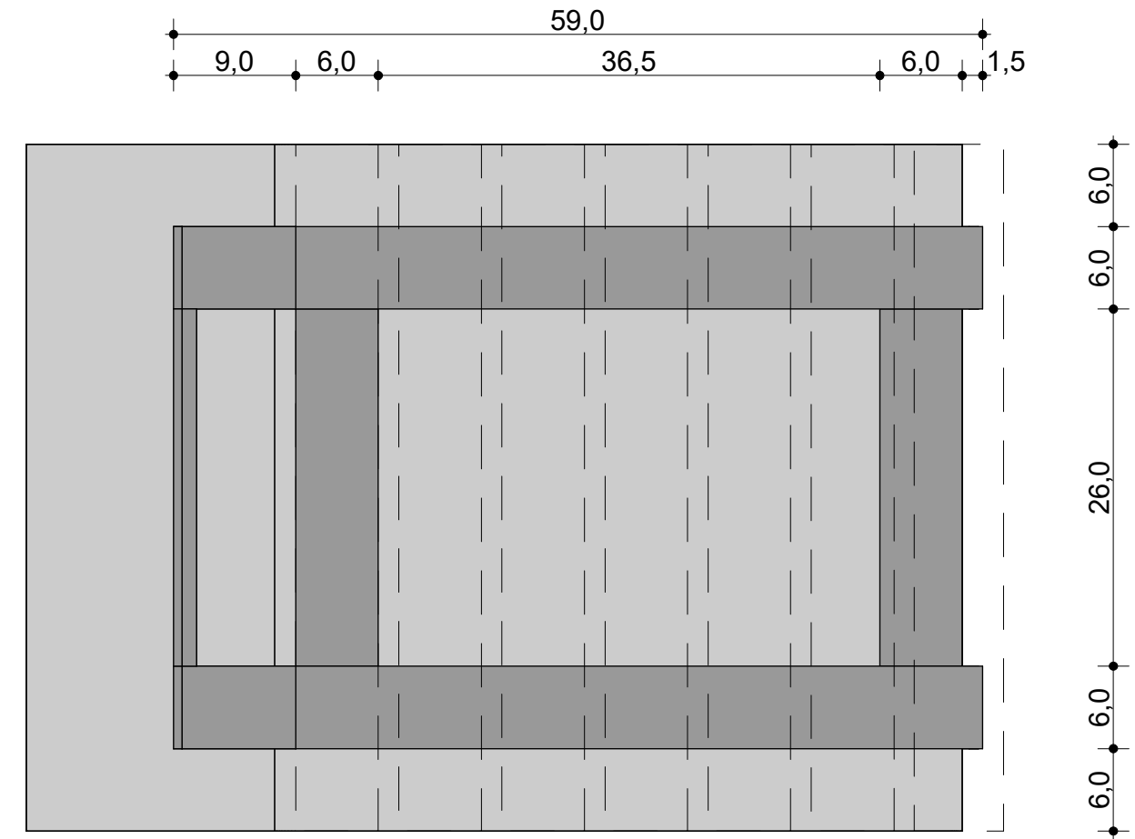
WIDOK Z GÓRY BEZ ODESKOWANIA
