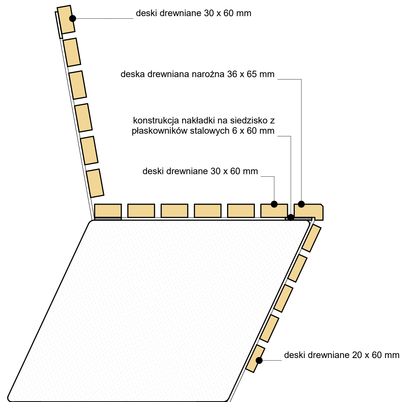
PRZEKRÓJ B-B
