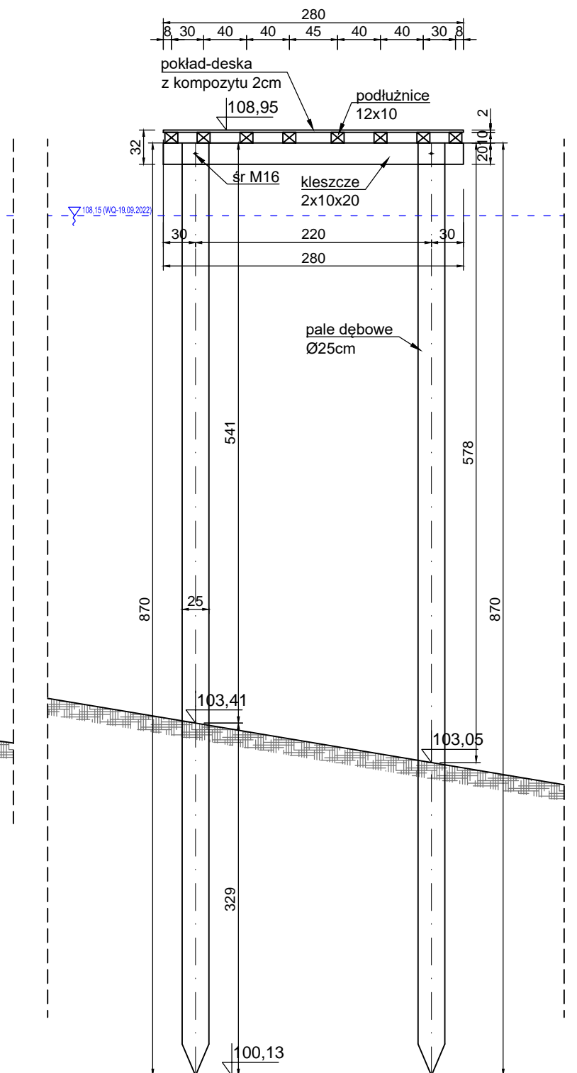
Przekrój D-D skala 1:50
