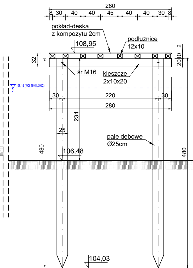
Przekrój B-B skala 1:50
