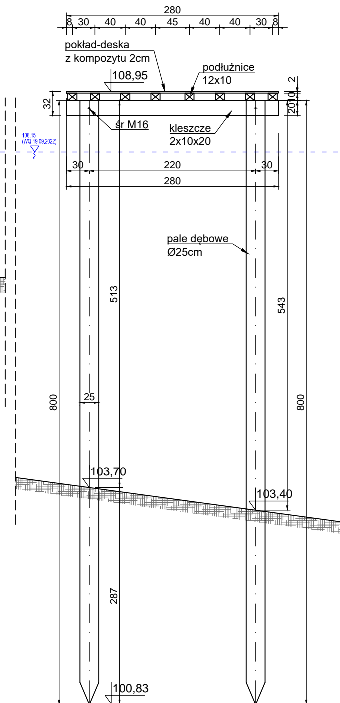
Przekrój C-C skala 1:50
