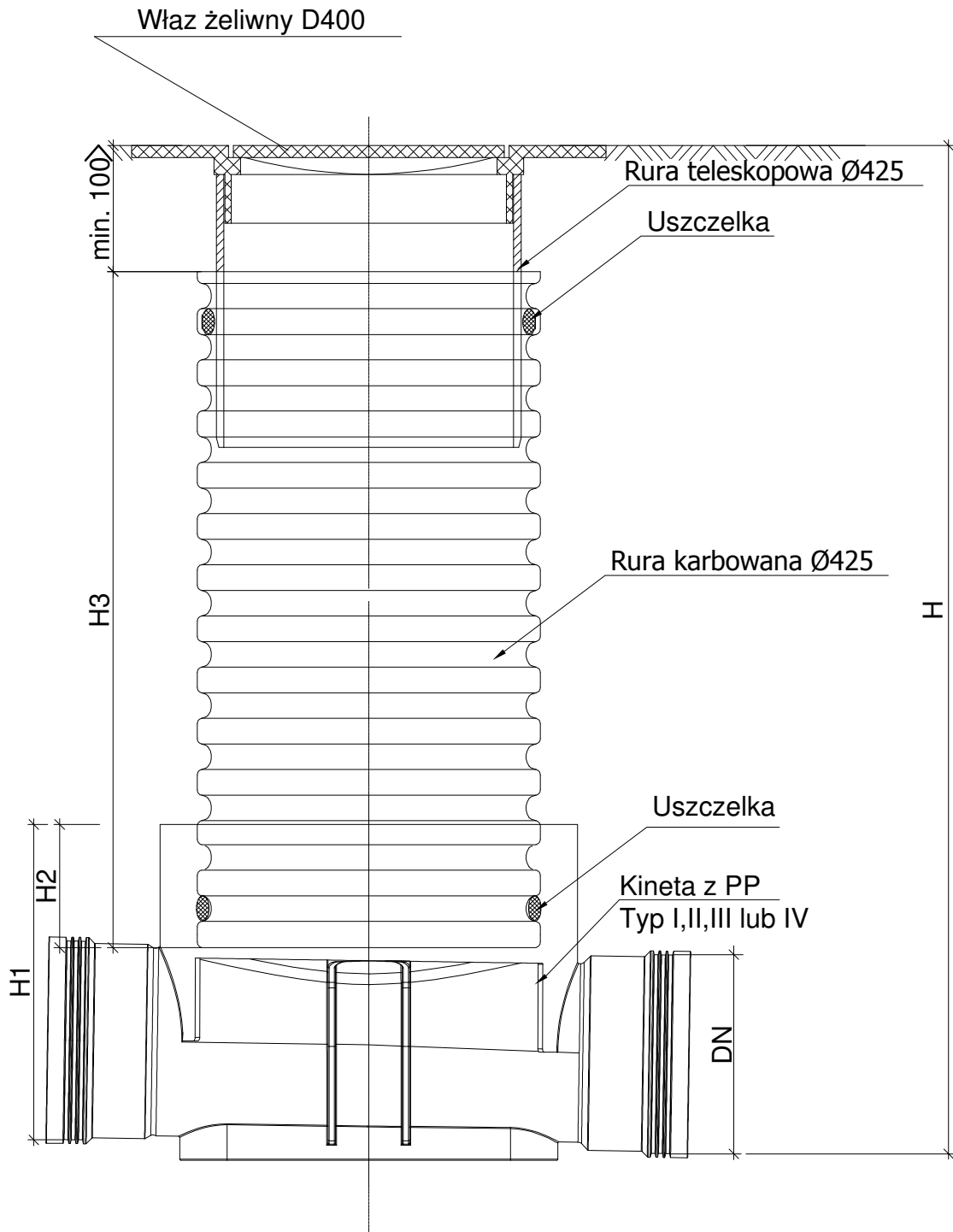
Studzienka kanalizacyjna Ø425 niewłazowa
