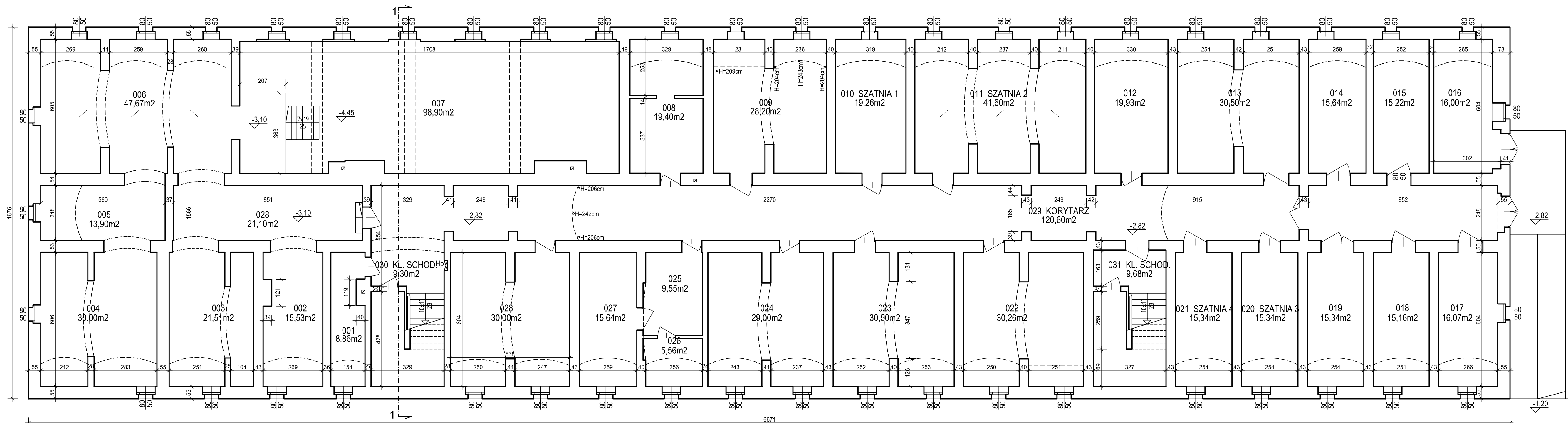
RZUT PIWNIC - STAN ISTNIEJĄCY 1:100 BUDYNEK "D"
