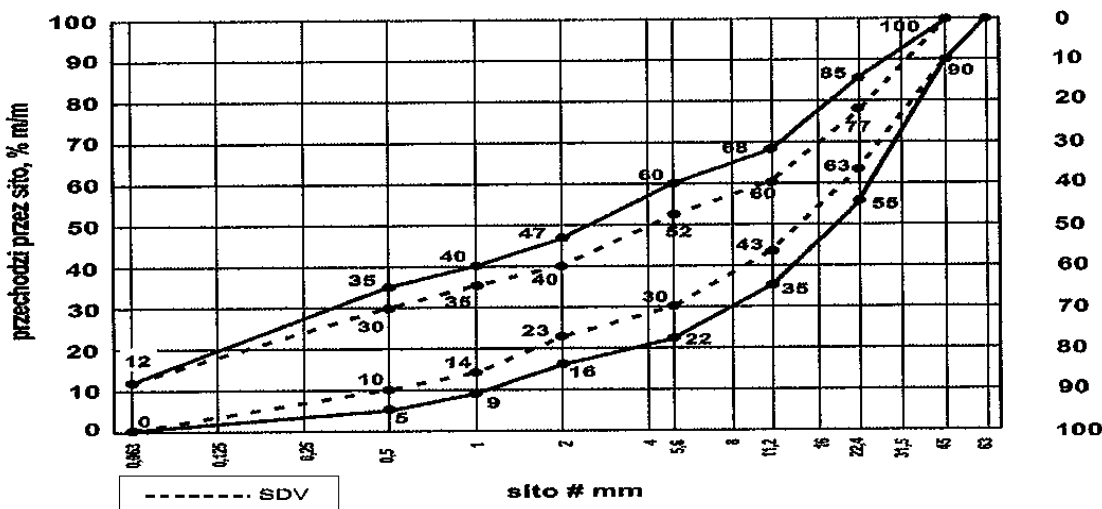
Rys. 2. Krzywe graniczne uziarnienia mieszanki kruszywa niezwiązanego 0/45 mm do warstw podbudowy
