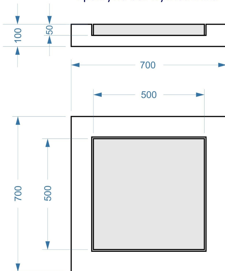
Rama pojedyncza i pokrywa bez wywietrznika
