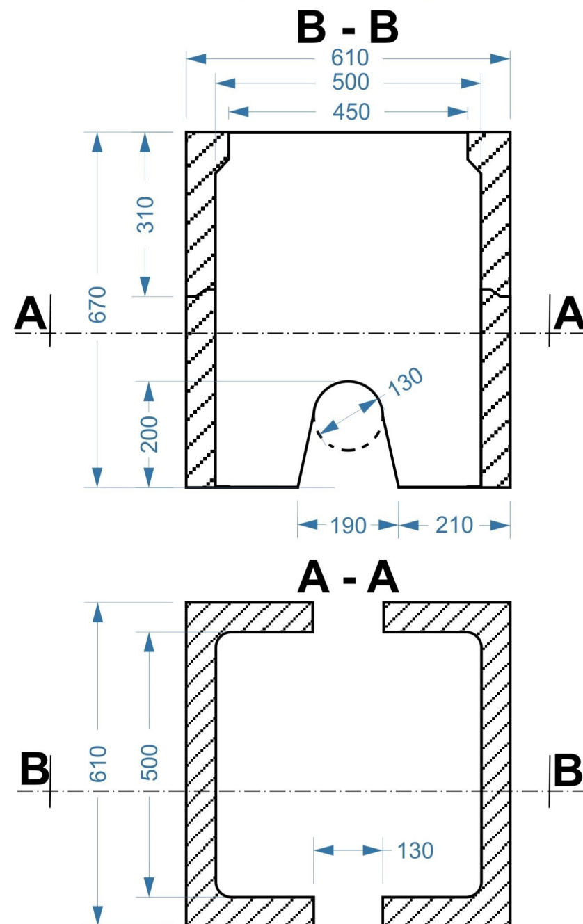
Korpus studzienki kablowej (dwuelementowy)
