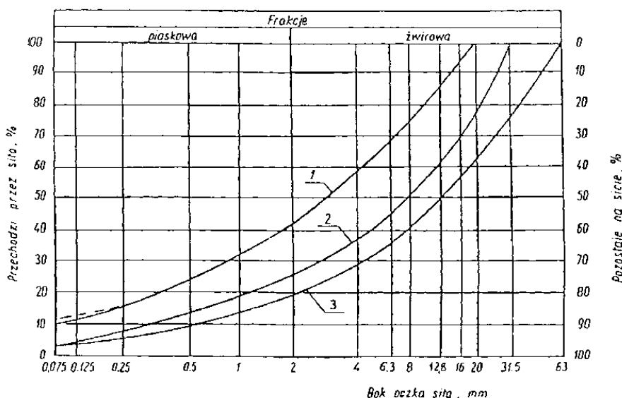
Rysunek 1. Pole dobrego uziarnienia kruszyw przeznaczonych na podbudowy wykonywane metodą stabilizacji mechanicznej 1-2 kruszywo na SRGEXGRZ JDVDGQLF] JyUQ ZDUVWZ OXE SRGEXGRZ MHGQRZDUVWZRZ 1- NUXVJ\ZR QD SRGEXGRZ SRPRFQLF] GROQ ZDUVWZ
