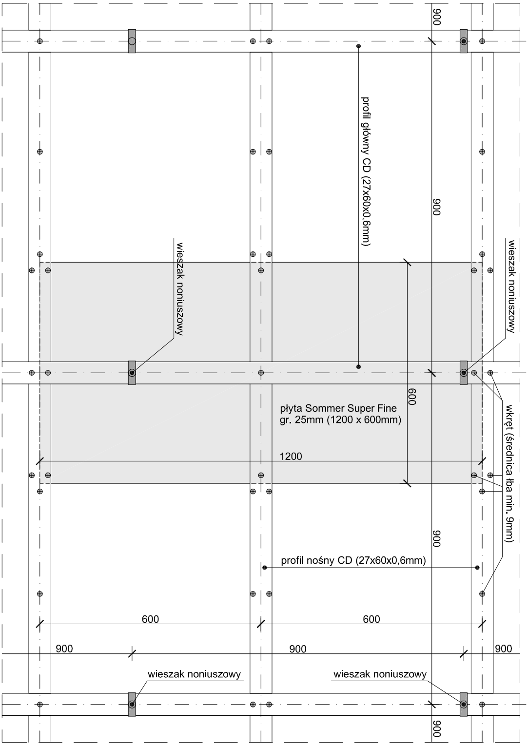
Rysunek elementu montażowego konstrukcji sufitu do użytku w hali sportowej "Sommer Super Fine" 25mm / profile CD
