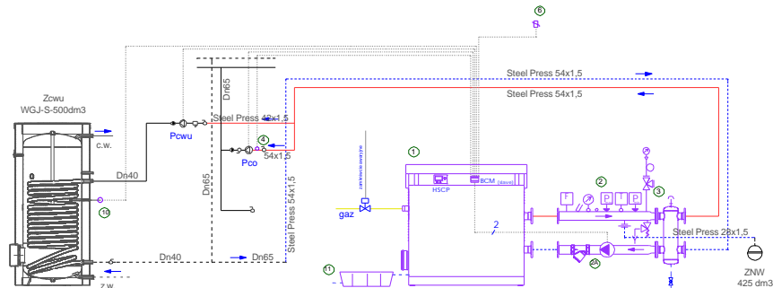
SCHEMAT TECHNOLOGICZNY KOTŁOWNI
