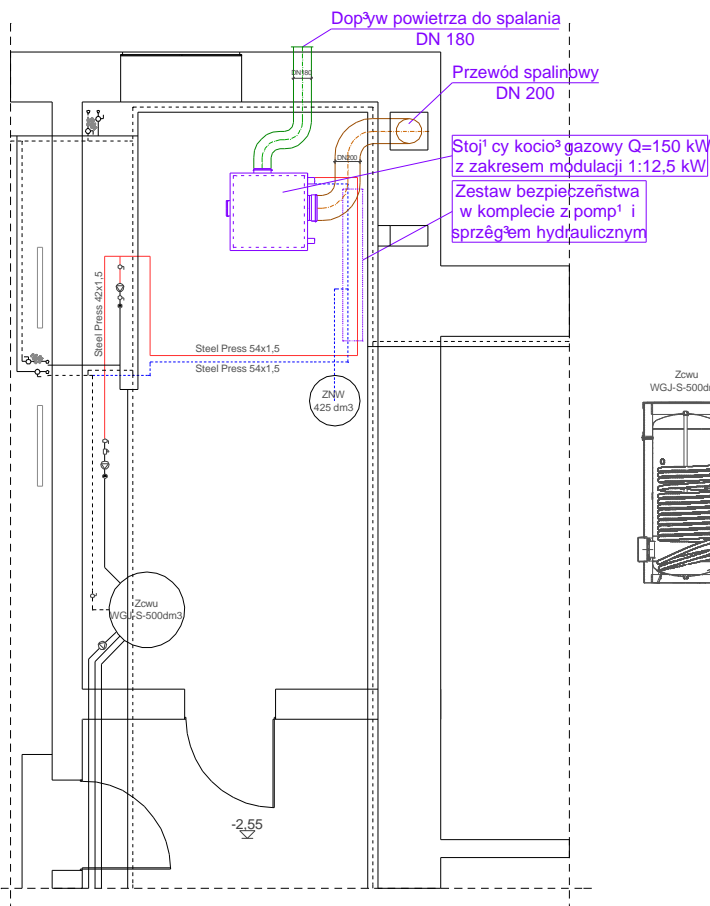
RZUT KOTŁOWNI skala - 1:25
