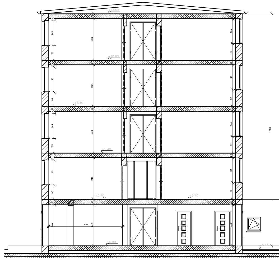
przekrój budynku A-A
