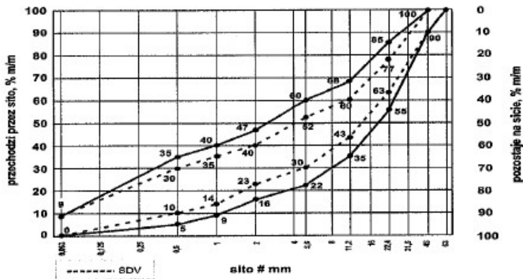
Rysunek nr 1 Uziarnienie mieszanki niezwiązanej 0/45 dla podbudowy zasadniczej
