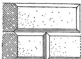
Fig.17 abgefaster Spiegel.
