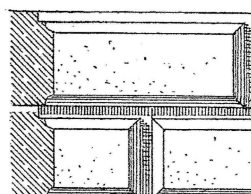
Fig 21 gekehiter Spiegel.
