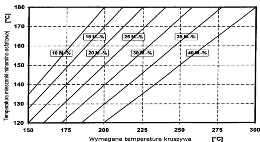
Tablica 13. Temperatura kruszywa w zależności od ilości zimnego i suchego granulatu asfaltowego
