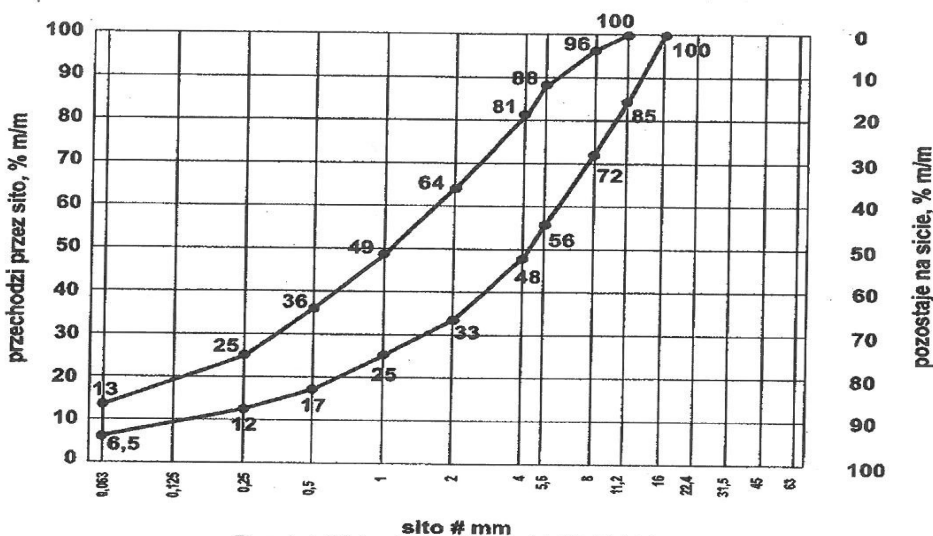
Rys. 1.4. Uziarnienie mieszanki CBGM 0/11,2
