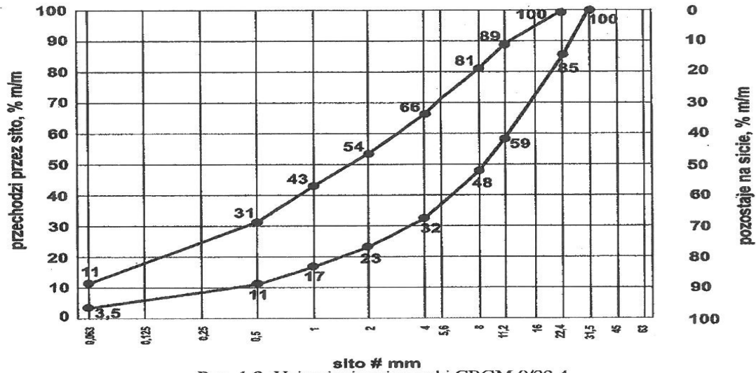
Rys. 1.2. Uziarnienie mieszanki CBGM 0/22,4
