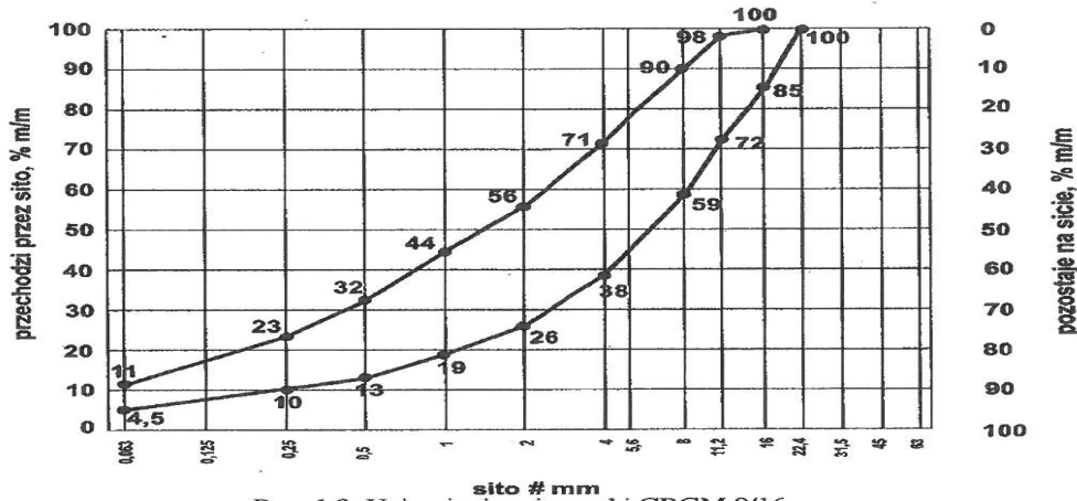
Rys. 1.3. Uziarnienie mieszanki CBGM 0/16
