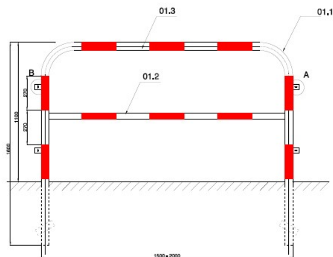
Rys. 1. Wzór bariery ochronnej z rur stalowych U-12a
