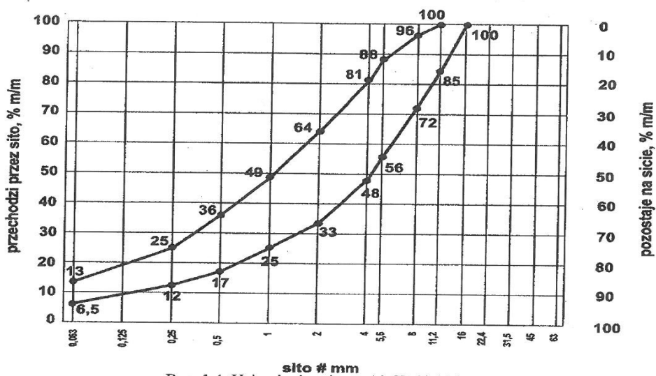
Rys. 1.4. Uziarnienie mieszanki CBGM 0/11,2
