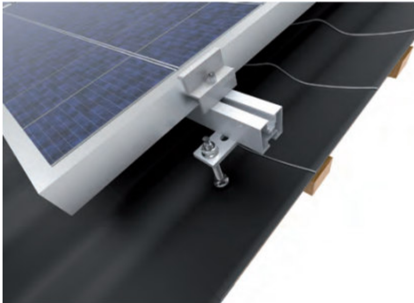
Rysunek 1. Przykład mocowania panelu fotowoltaicznego na dachu.
