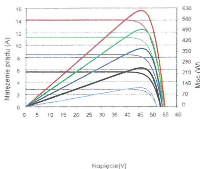
Krzywe prądowo-napięciowe i mocowo-napięciowe (615 Wp)
