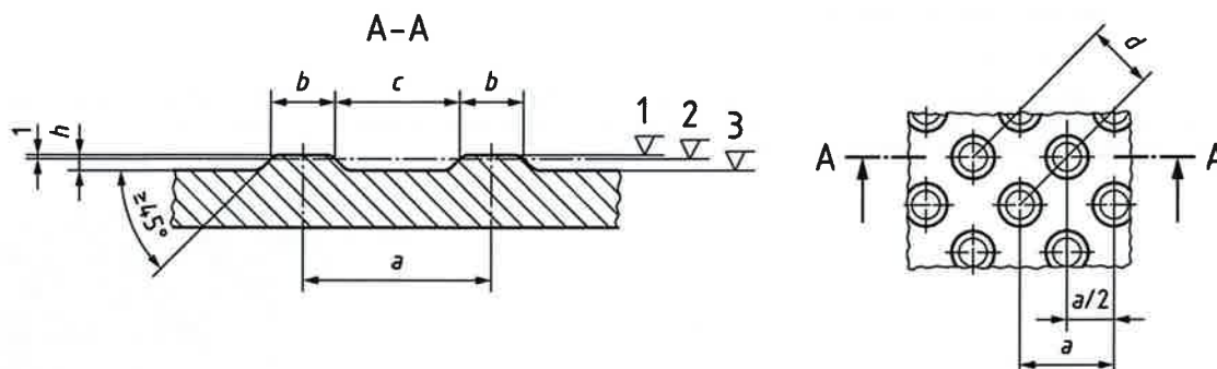
a = 58-60 mm, b = 20-22 mm, c = 37-39 mm, d = 40-42 mm, h=4.5+5 mm i (przy tolerancji 0.5mm) zawsze h \geq 4.5 mm Rys 2b. Wymiary wypustek płytki ostrzegawczej na podstawie normy DIN 32984
