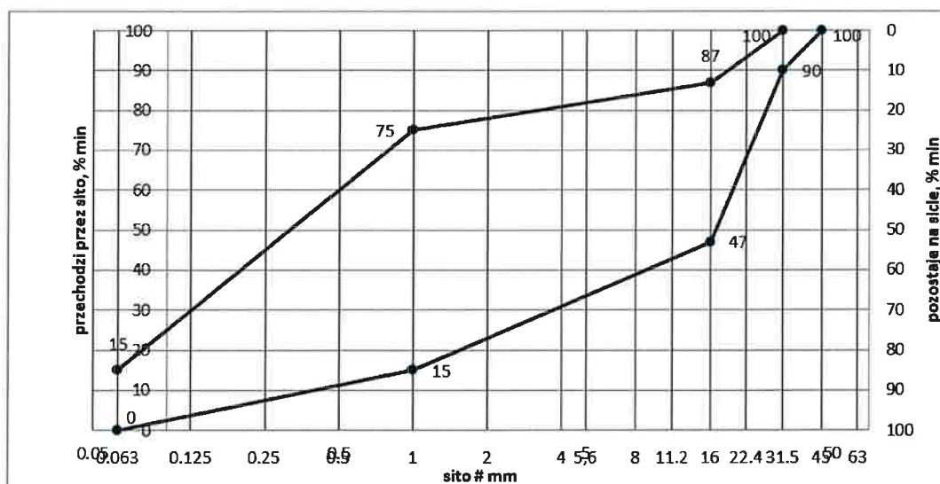
Rysunek 1. Mieszanka niezwiązana 0/31,5 do warstwy ulepszonego podłoża stabilizowanego georusztem
