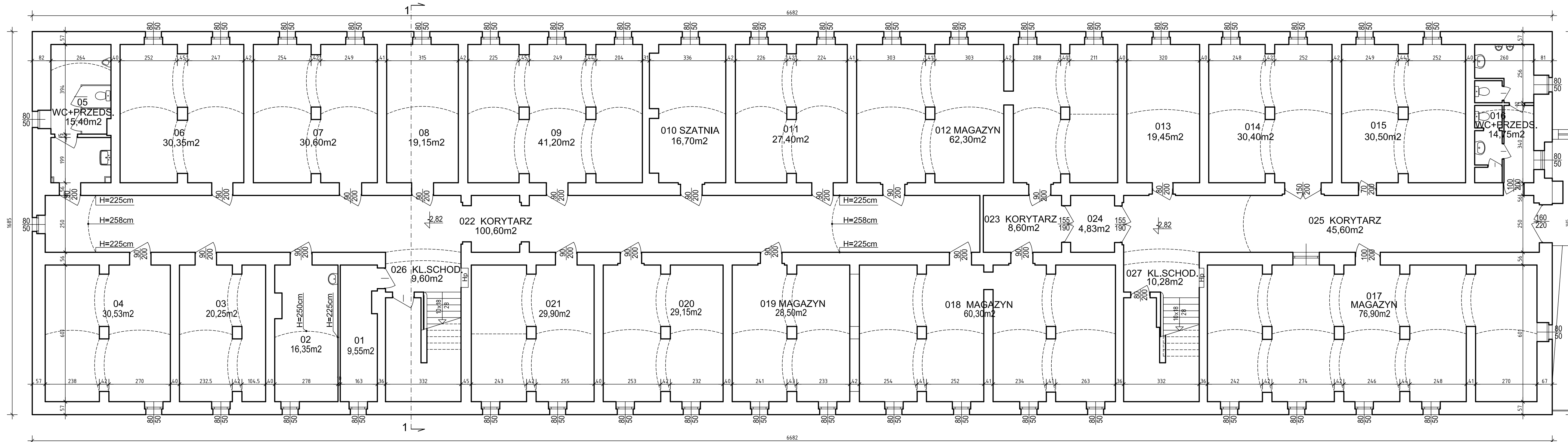
RZUT PIWNIC - STAN ISTNIEJĄCY 1:100 BUDYNEK "B"
