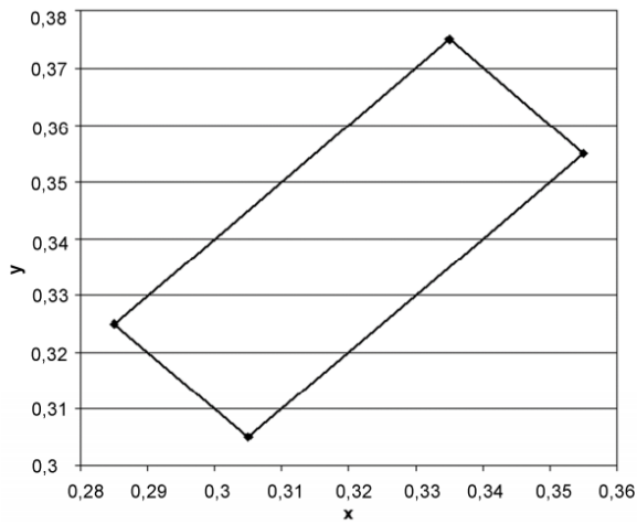
Rys. 1. Współrzędne chromaticzności x,y dla barwy białej oznakowania
