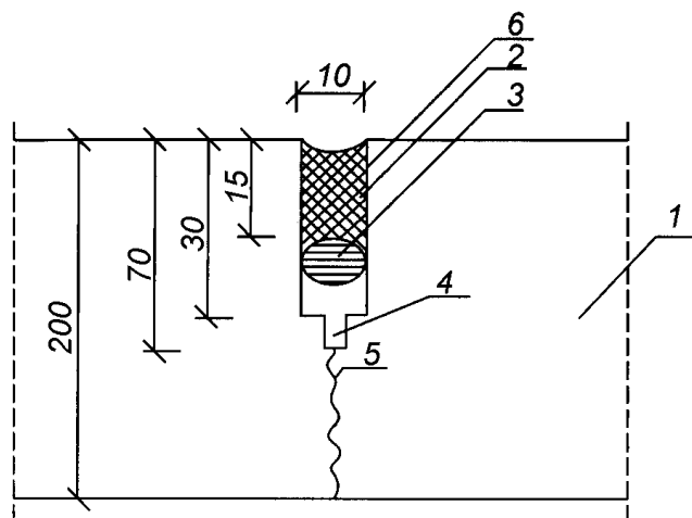
Rys. Przykład uszczelnienia szczeliny skurczowej pozornej w podbudowie z betonu cementowego 1-płyta betonowa, 2-masa uszczelniająca, 3-sznur uszczelniający, 4-wstępne nacięcie szer. 3 mm, 5-pęknięcie powierzchni wskutek skurczu, 6-zagруntowanie bocznych ścianek roztworem gruntującym
