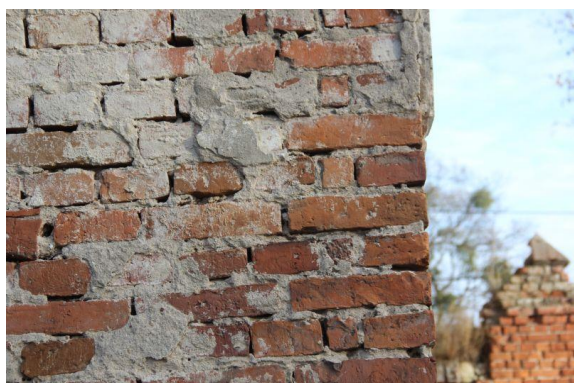
Fot. 10-15. Zdjęcia spichrza obrazujące sposób wymurowania.
