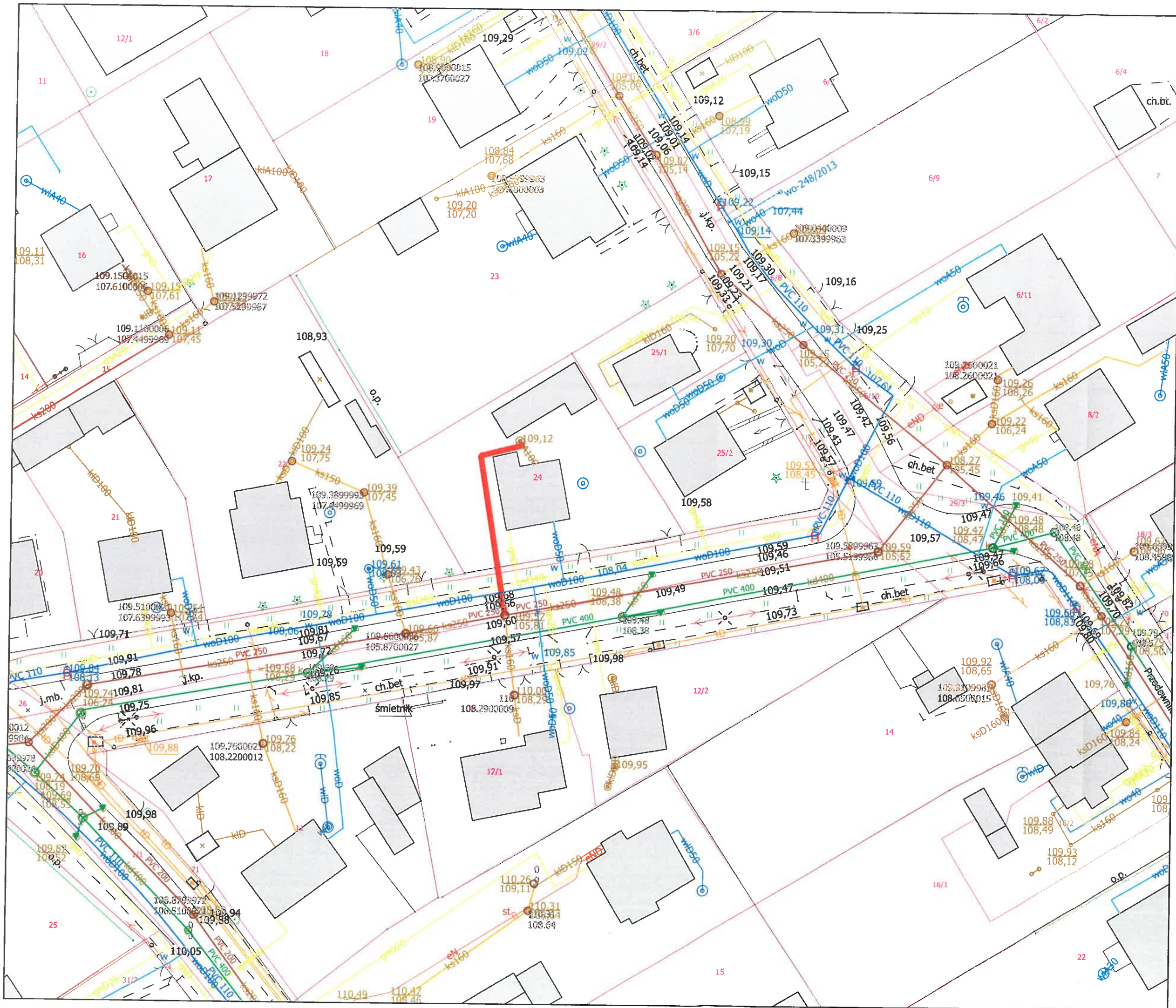
Przyłącze kanalizacji sanitarnej Adres: ul. Sikorskiego 4 Grodzisk Mazowiecki dz. nr ew. 24 obręb 60
