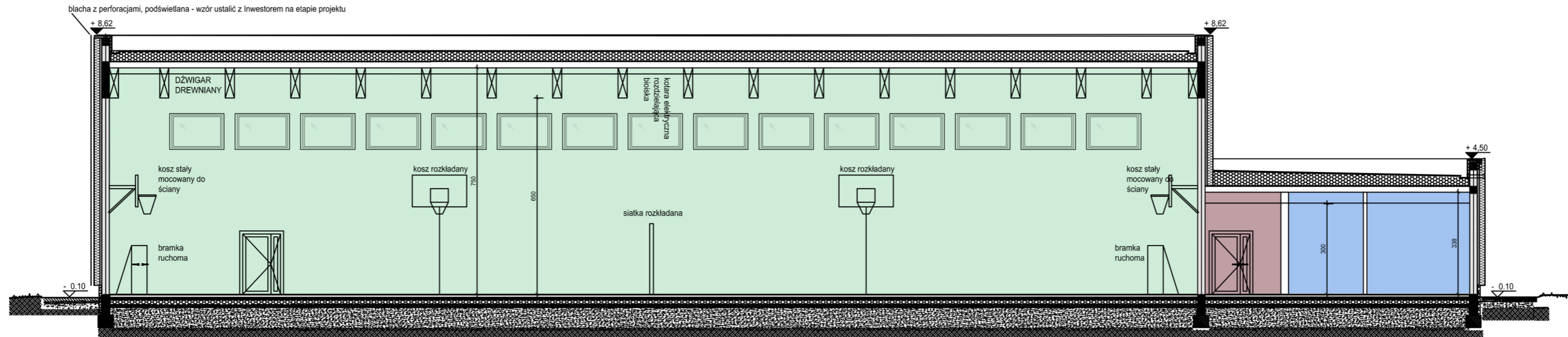
PRZEKRÓJ AA
