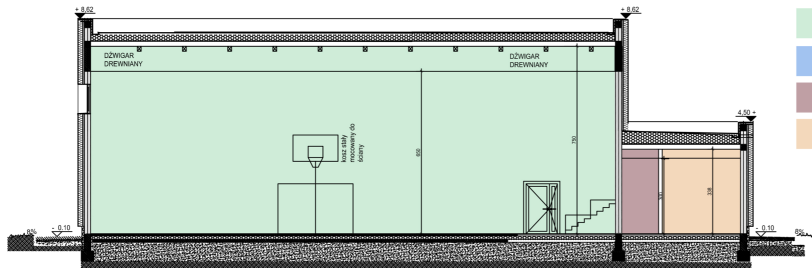
PRZEKRÓJ BB
