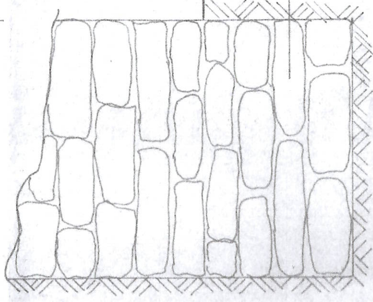
Odkrywka fundamentu Nr 3
