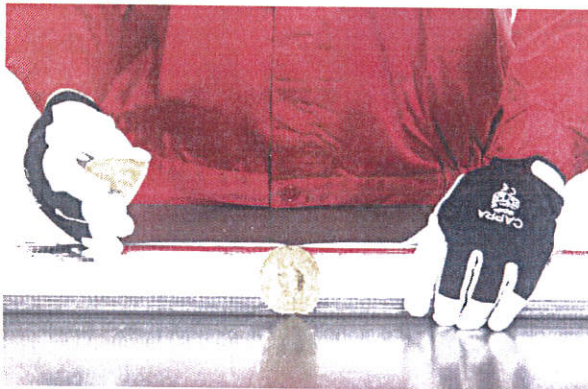
Wycięcie klina 2 \times 45^\circ w odcinku prostym, w miejscu trójnika.
