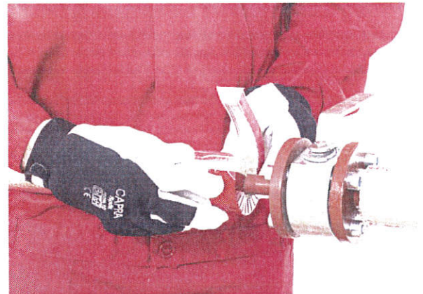
Zabezpieczenie zakończenia odcinka prostego izolacji przy zaworze mankietem aluminiowym.
