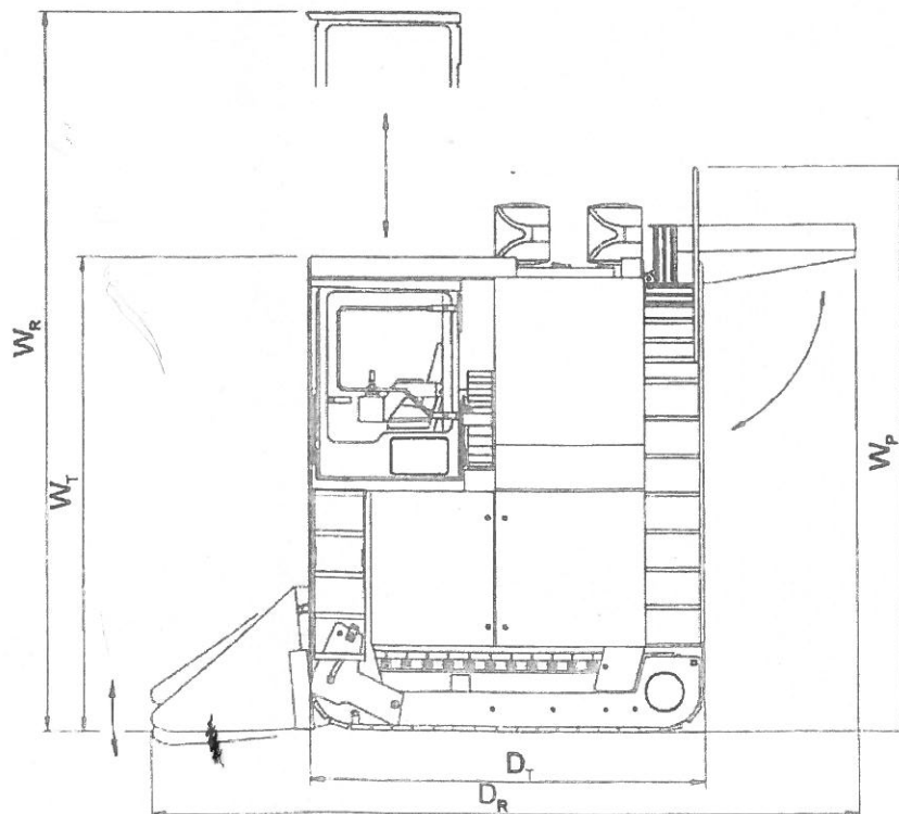
Rysunek 8-2: Wymiary maszyny
