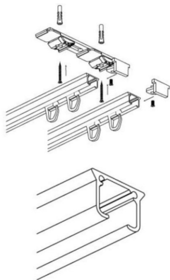
SYSTEM KARNISZOWY ZS2 CREATIVA
