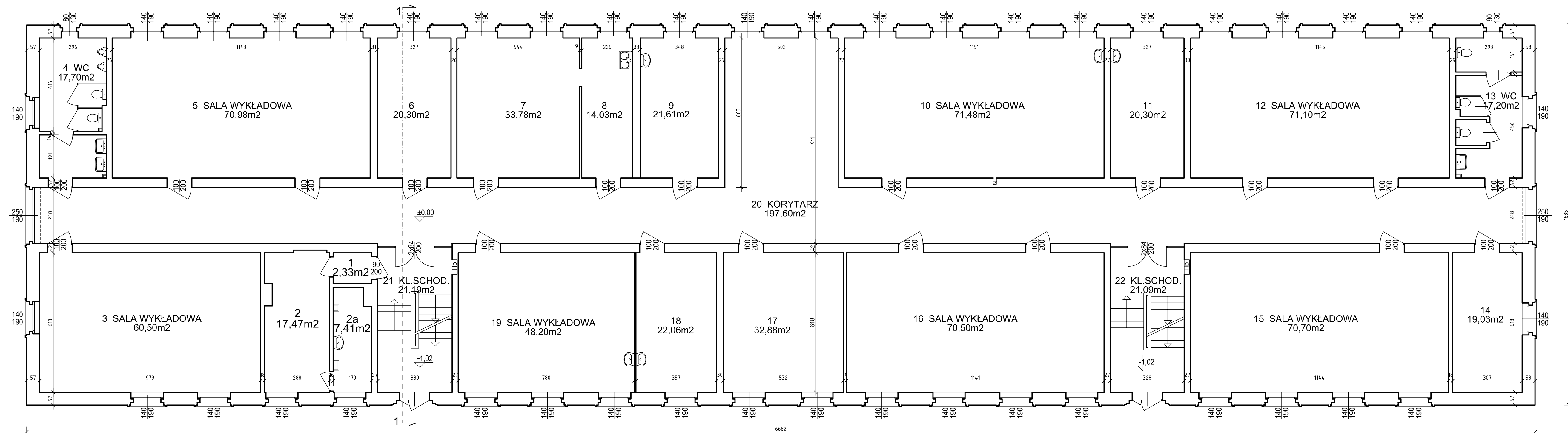
RZUT PARTERU - STAN ISTNIEJĄCY 1:100 BUDYNEK "B"
