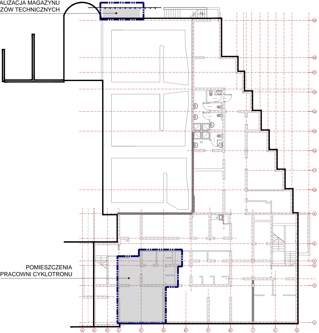
RZUT PIWNIC BUDYNKU PET
