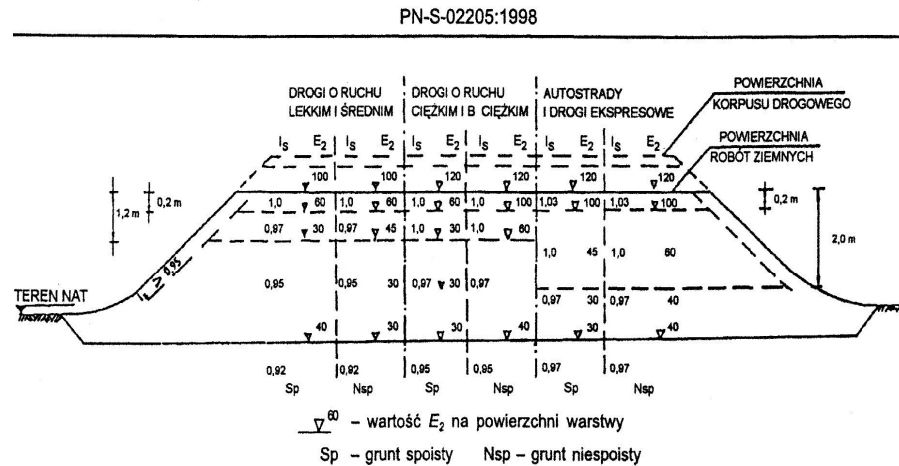
Rysunek 3 – Wartości wymagane w nasypach: wskaźnika zagęszczenia I_s i wórnego modułu odkształcenia E_2 , megapaskali
