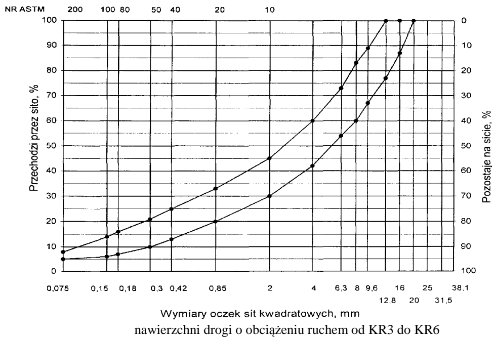
Rys. 13. Krzywe graniczne uziarnienia mieszanki mineralnej BA od 0 do 16 mm do warstwy wyrównawczej
