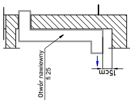
Szegół wentylacji - schemat
