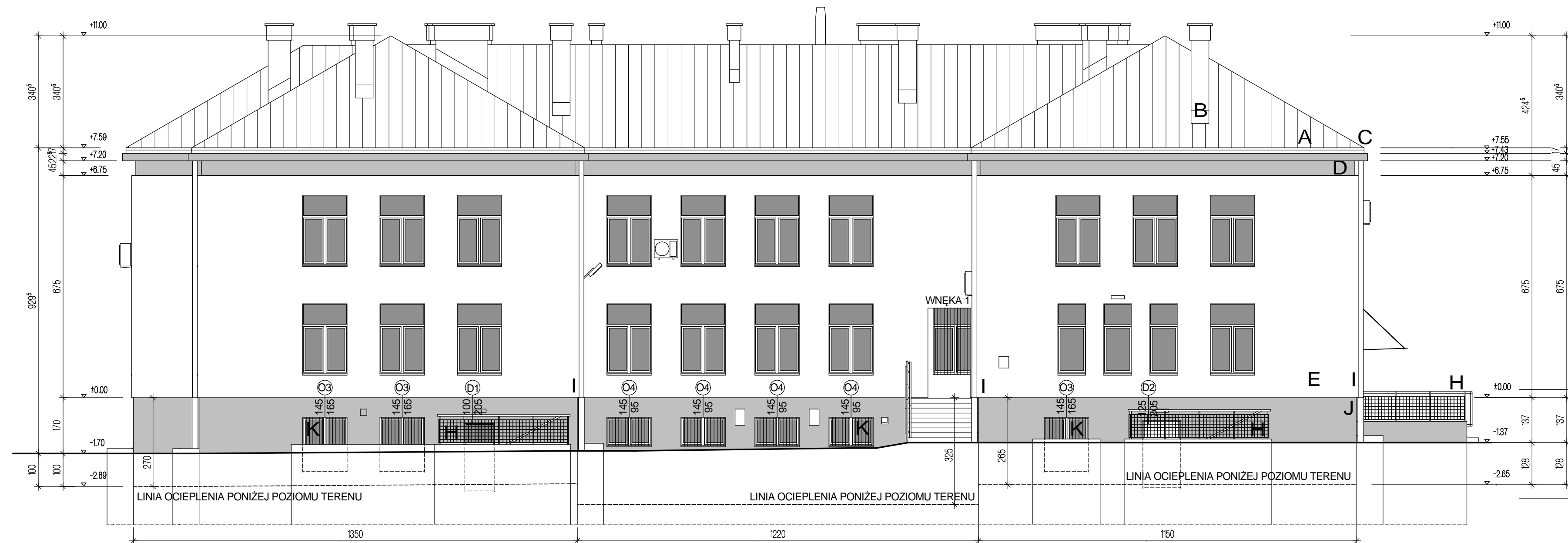
ELEWACJA WSCHODNIA
