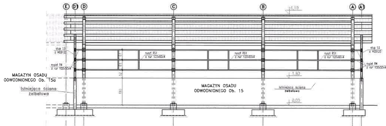
Konstrukcja ryglowa w osi 2-2
