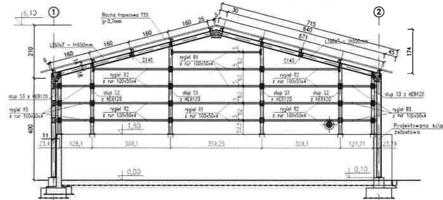
Konstrukcja ryglowa w osi A1 | D1 (w osi D1 wykonanie w lustrzanym odbiciu)
