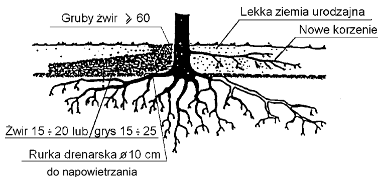
Rys. 2. Pień drzewa obsypany na wysokość 0,2 - 0,5 m ze specjalnymi napowietrzającymi warstwami żwirowymi
