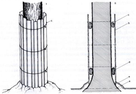
Rys. A – Sposób oszalowania pni drzew (rys. Z. Chachulski, Chirurgia i pielęgnacja drzew, Józefów-Michalin, 2000)
