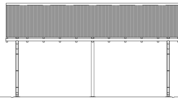
ELEWACJA 1:50
