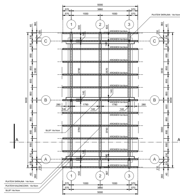
Wszystkie wymiary podano w mm. KONSTRUKCJA GŁÓWNA - RZUT WIEŻBY DACHOWEJ 1:50
