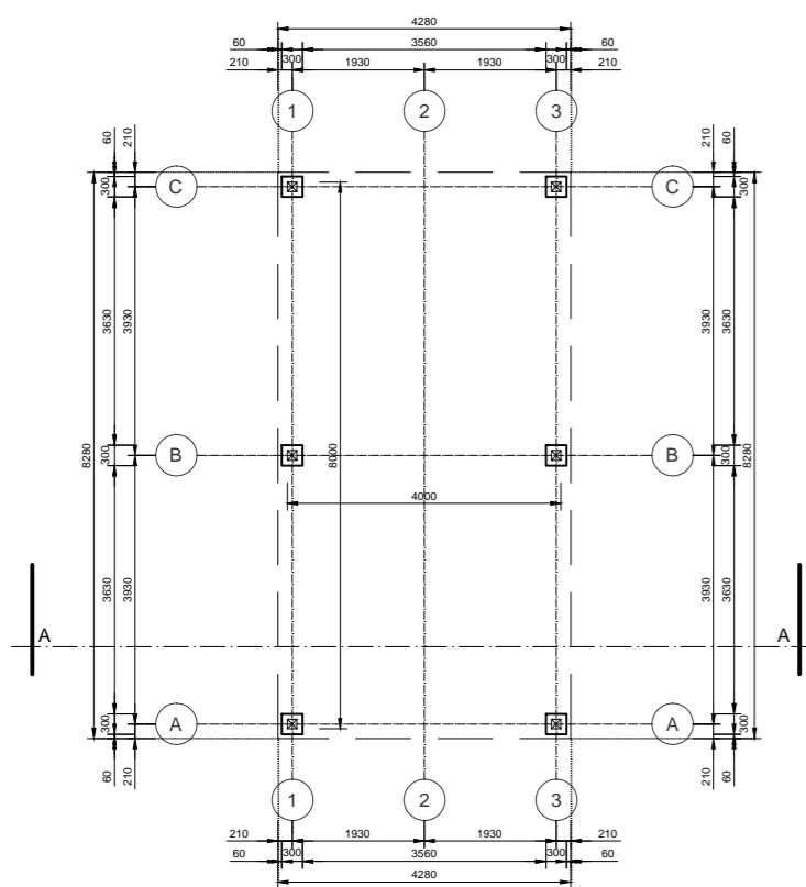
Wszystkie wymiary podano w mm. KONSTRUKCJA GŁÓWNA - RZUT FUNDAMENTÓW 1:50
