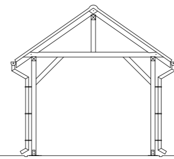
ELEWACJA 1:50
