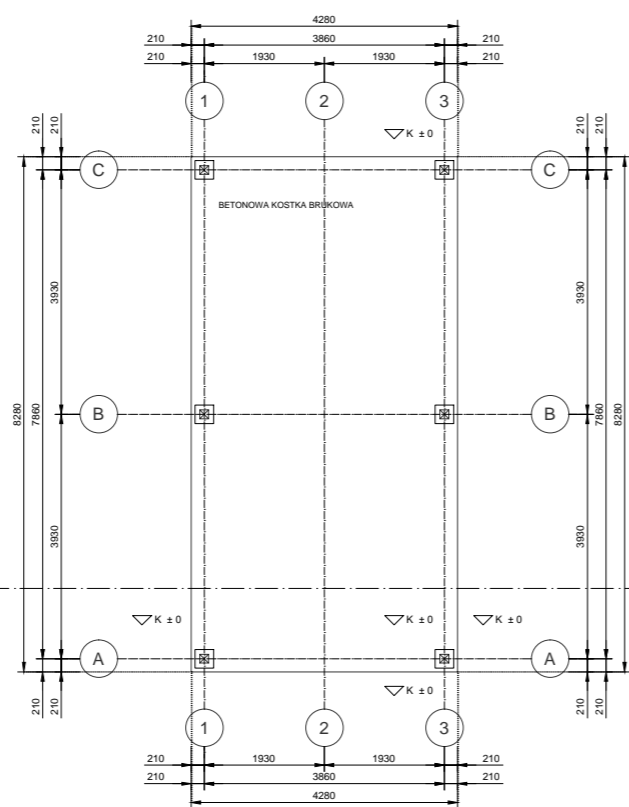
Wszystkie wymiary podano w mm. KONSTRUKCJA GŁÓWNA - RZUT PRZYZIEMIA 1:50
