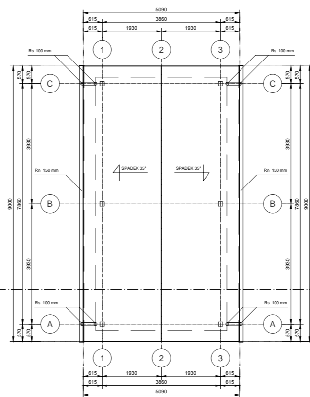
Wszystkie wymiary podano w mm. KONSTRUKCJA GŁÓWNA - RZUT DACHU 1:50
