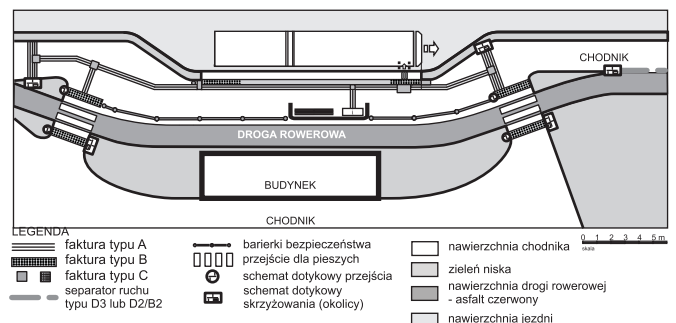
Ryc. 6.4. Przykład rozwiązania przebiegu drogi rowerowej i dojść pieszych w obrębie przystanku komunikacji miejskiej. (źródło: Wysocki 2010, s.132)
