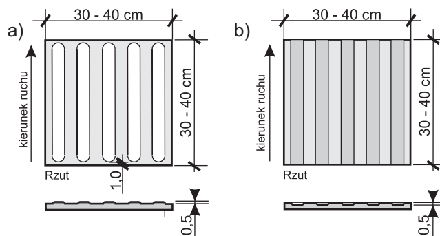
Ryc. 2.6. Płytki kierunkowe do zastosowań: a) na zewnątrz i wewnątrz obiektów, b) do wewnątrz i zadanych peronów zewnętrznych. (oprac. autora na podstawie BS 8300, 2000).
