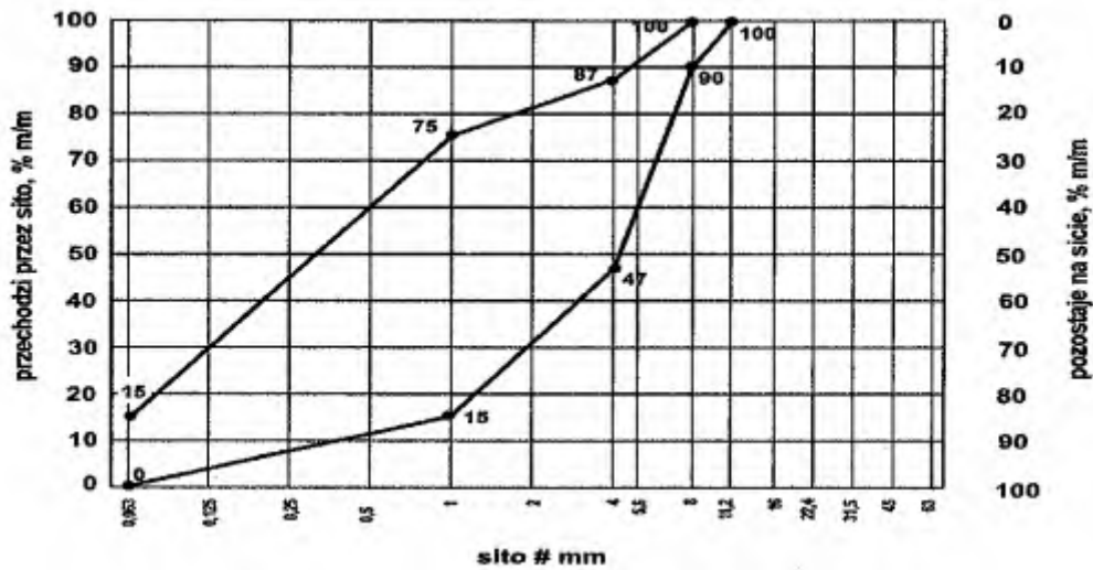
Rys. 2. Uziarnienie mieszanki niezwiązanej 0/11,2 do warstwy mrozochronnej/odsączającej
