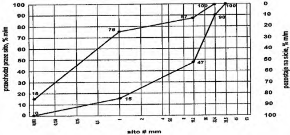
Rys. 4. Uziarnienie mieszanki niezwiązanej 0/22,4 do warstwy mrozochronnej/odsączającej.
