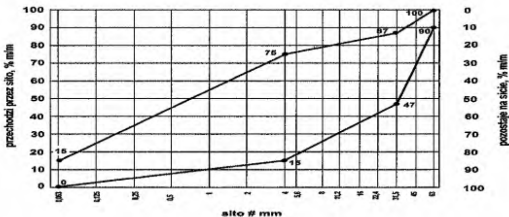
Rys. 7. Uziarnienie mieszanki niezwiązanej 0/63 do warstwy mrozochronnej/odsączającej
