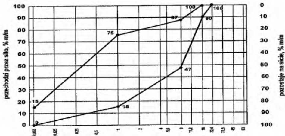
Rys. 3. Uziarnienie mieszanki niezwiązanej 0/16 do warstwy mrozochronnej/odsączającej
