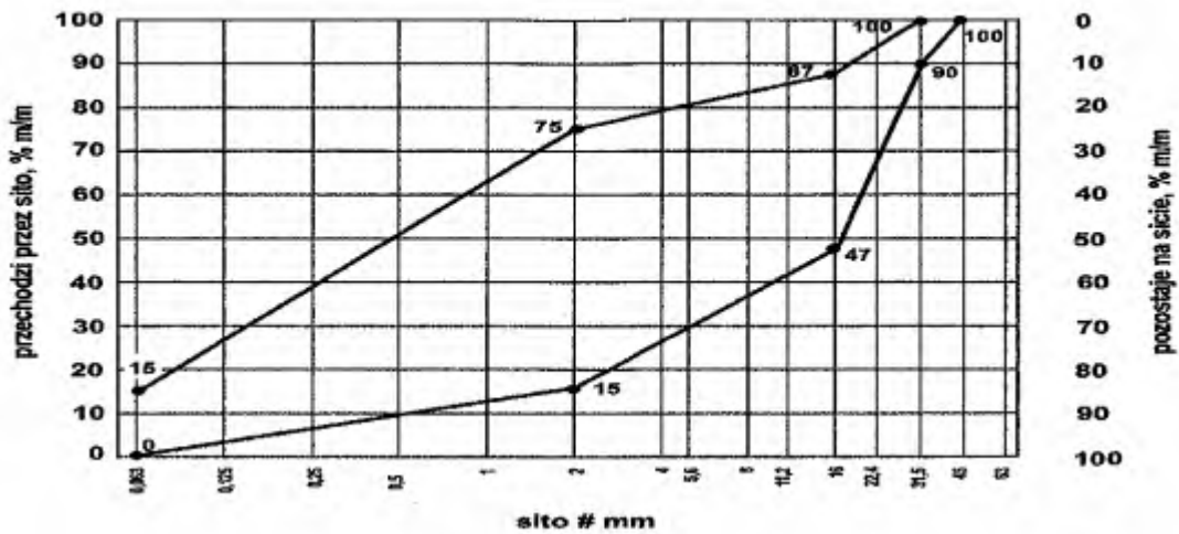
Rys.6. Uziarnienie mieszanki niezwiązanej 0/45 do warstwy mrozochronnej/odsączającej
