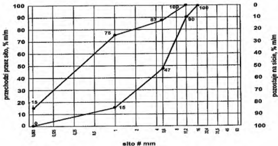
Rys. 3. Uziarnienie mieszanki niezwiązanej 0/16 do warstwy mrozochronnej/odsączającej
