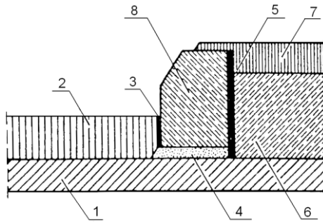
Rys. 4.1. Przykład wykonania krawężnika: 1- warstwa wiążąca, 2 - warstwa ścieralna, 3 - samoprzylepna taśma uszczelniająca połączenie warstwy ścieralnej z krawężnikiem, 4 - masa zalewowa pod krawężnik z mieszanki mineralno-asfaltowej, 5 - masa zalewowa w złączeniu podłużnym, 6 - płyta betonowa, 7 - warstwa ścieralna z asfaltu lanego na chodniku, 8 - krawężnik kamienny
