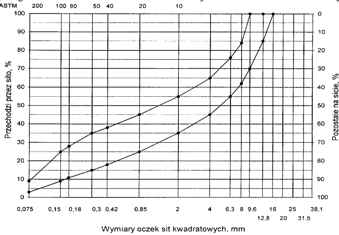
Rys. 10. Krzywe graniczne uziarnienia mieszanki mineralnej BA od 0 do 12,8 mm do warstwy wiążącej, wyrównawczej i wzmocniającej nawierzchni drogi o obciążeniu ruchem KR1 lub KR2
