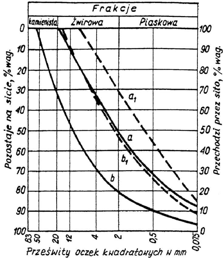
Rysunek – Obszar uziarnienia optymalnych mieszanek żwirowych
