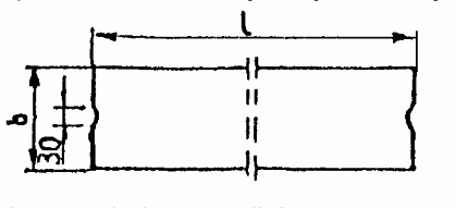
Rys. 1. Wymiarowanie krawężników
