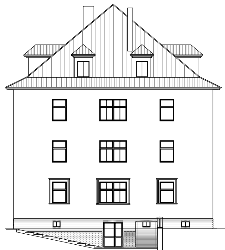
ELEWACJA PÓLNOCNA
