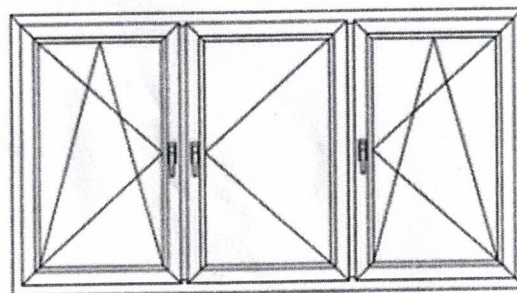
Okno trójskrzydłowe rozwierno-uchylne / rozwiernie / rozwierno-uchylne
