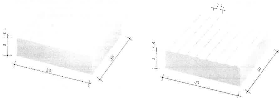
a) płytki ostrzegawcze (z wypustkami) b) płytki kierunkowe (rowkowane) symetryczne
