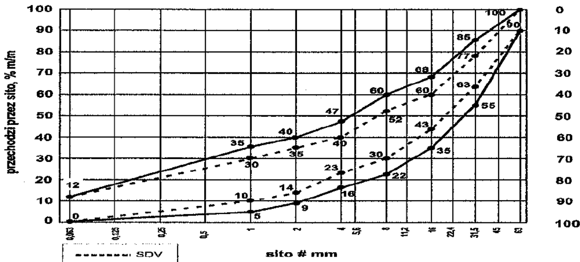
Rysunek 2. Uziarnienie mieszanki niezwiązanej 0/63 do podbudowy pomocniczej
