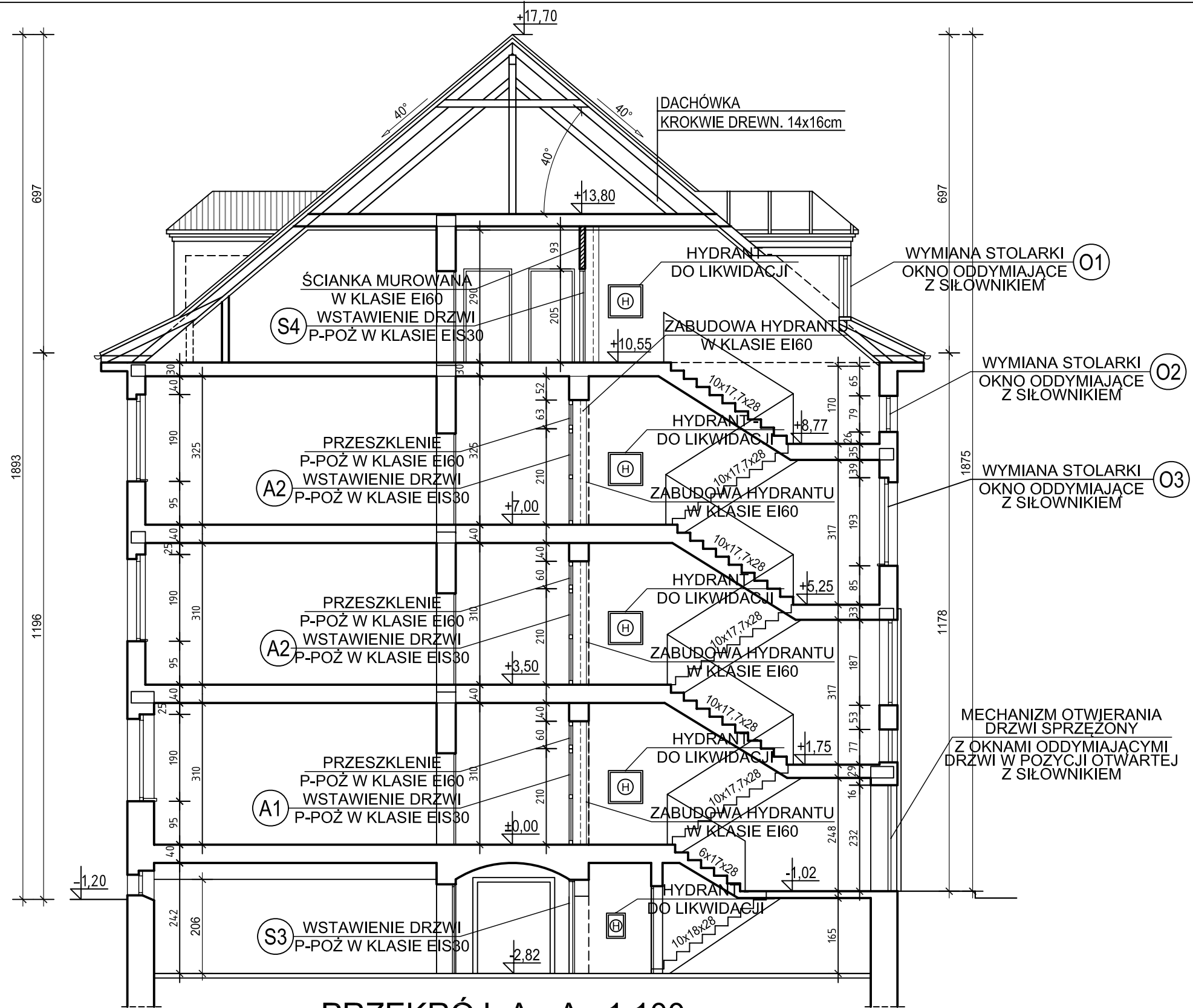
PRZEKRÓJ A - A 1:100 BUDYNEK "D"
