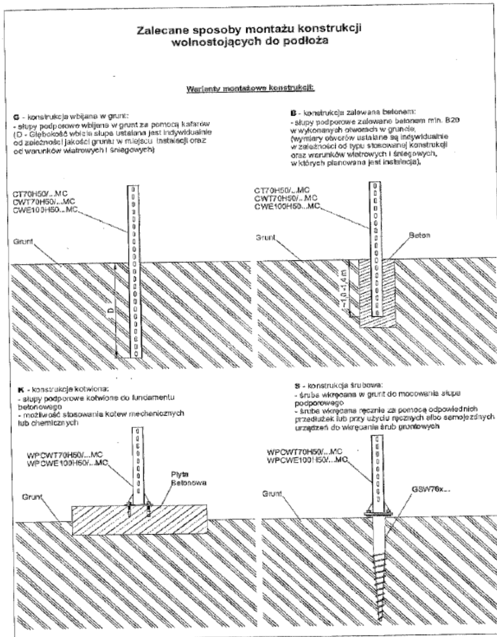
Rysunek 3. Sposoby montażu konstrukcji do podłoża.
